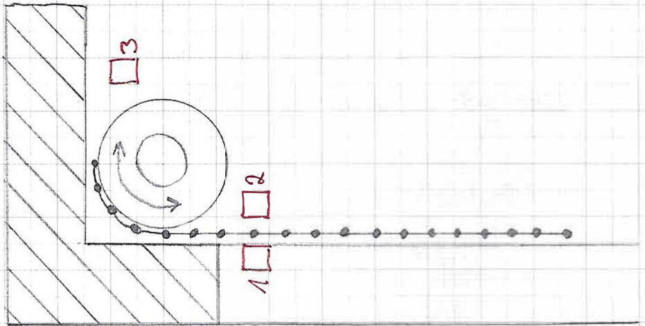
Rollgittertor
